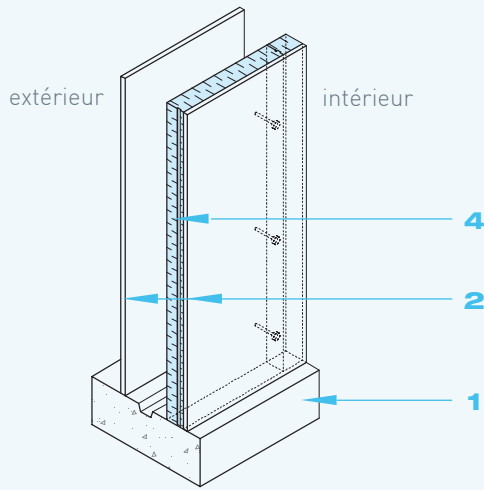
INSTALLATION INTÉRIEURE
