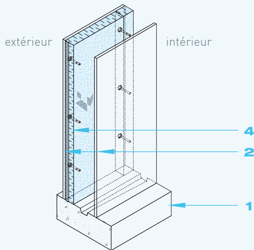
INSTALLATION EXTÉRIEURE
