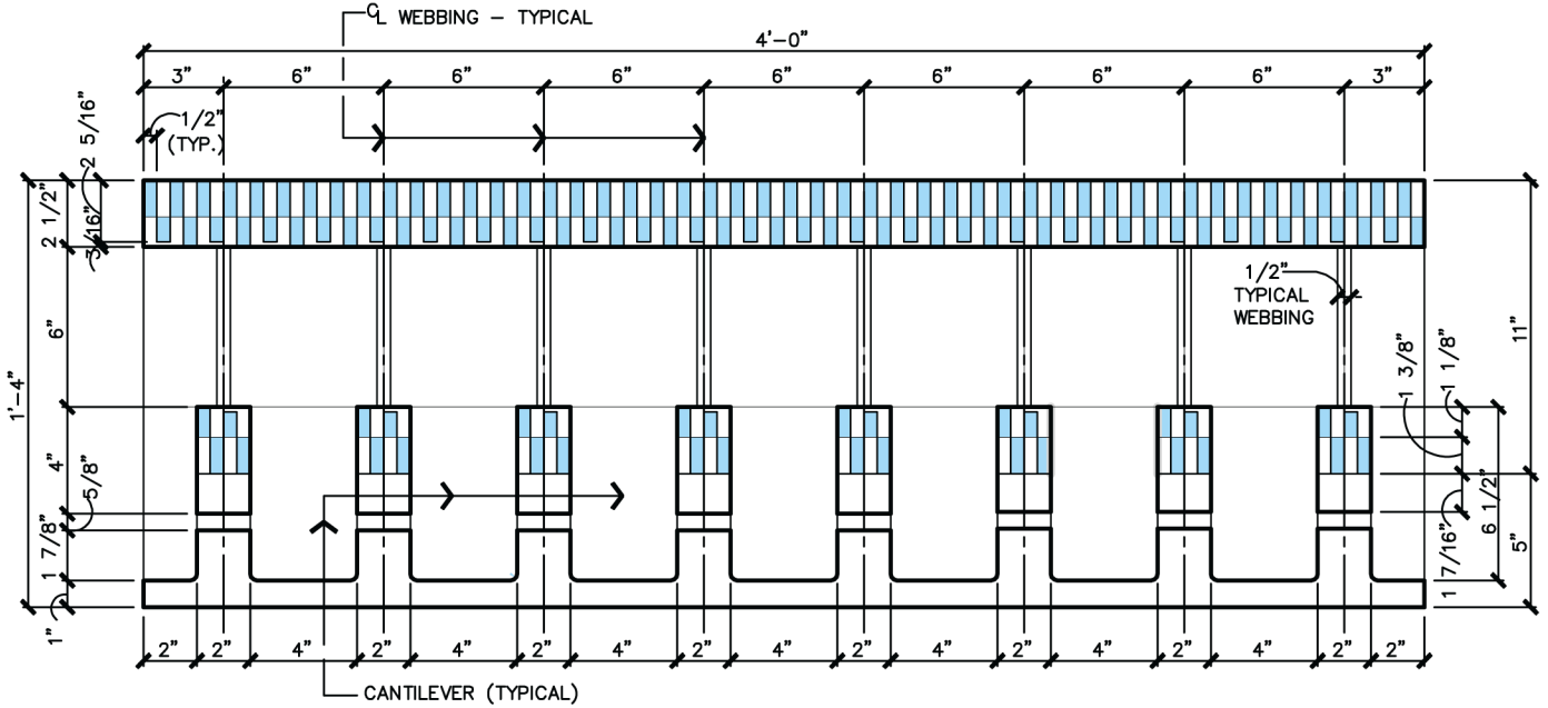
2 TOP VIEW SCALE: 1 1/2" = 1'-0"
