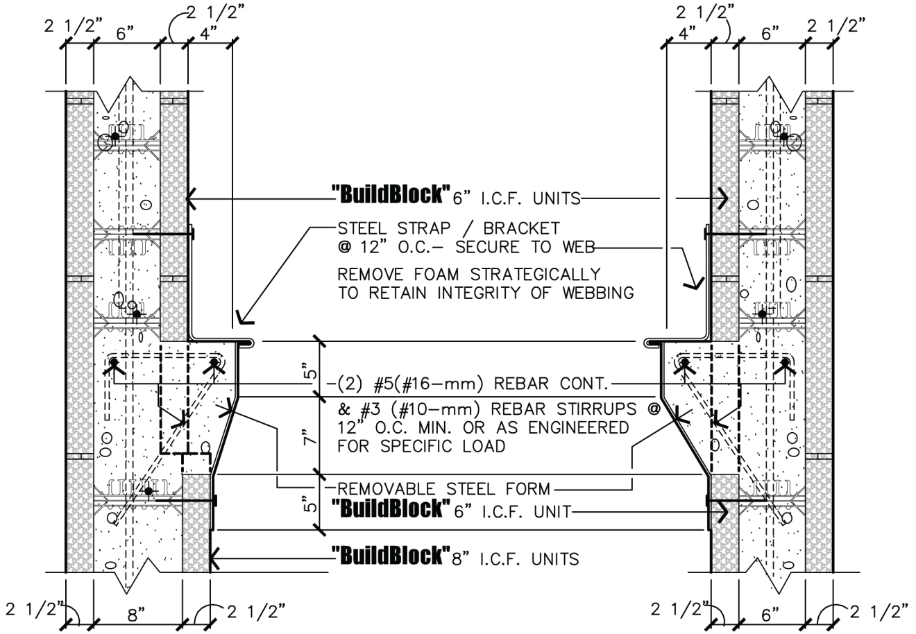
2 SECTION DETAIL SCALE: 1" = 1'-0"
