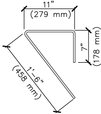
3 STIRRUP DETAIL SCALE: 1" = 1'-0"
